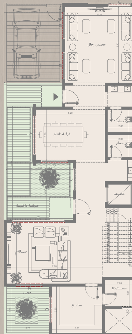
مخطط الطابق الأرضي
